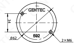
底座安装
